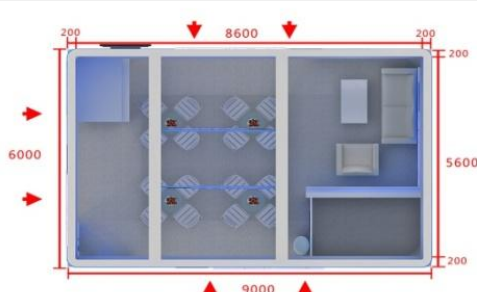
平面布置图
