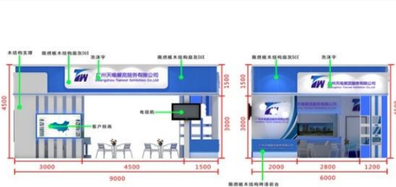
正面立面图
